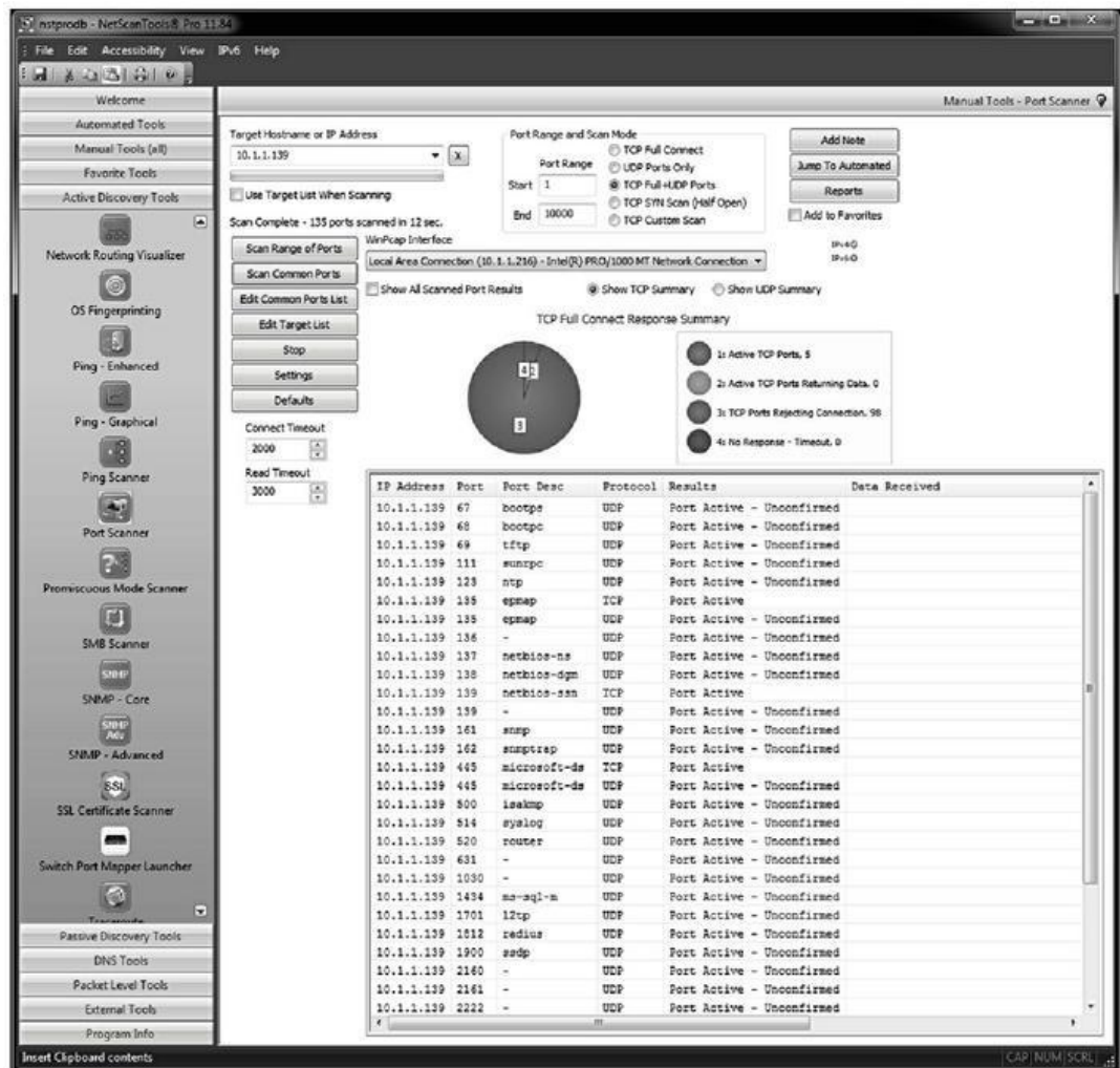
Figure 12.1 : Analyse des ports d'une machine Windows 10 avec NetScanTools Pro.
