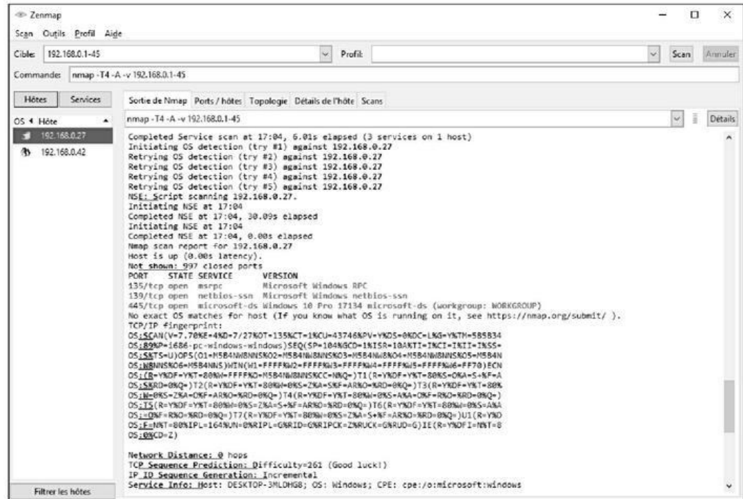
Figure 9.1 : Résultat d'un balayage sweep d'un réseau en classe C avec Nmap
