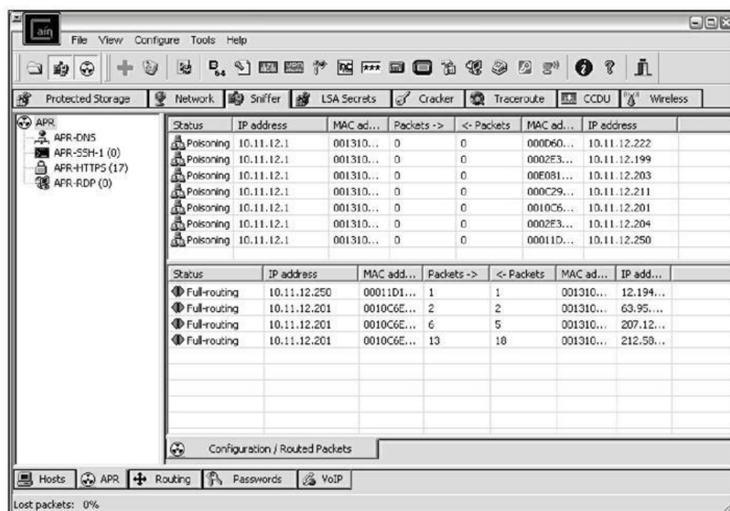
Figure 9.12 : Résultat d'un empoisonnement ARP avec Cain & Abel.
