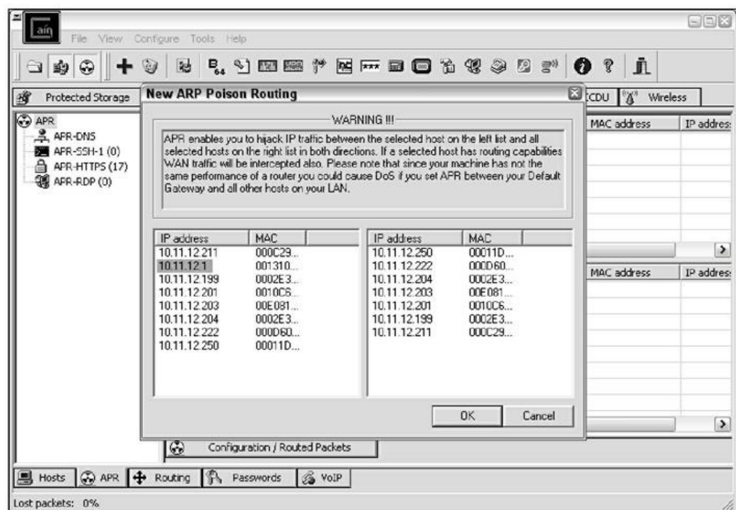
Figure 9.11 : Sélection des victimes de l'empoisonnement ARP dans Cain & Abel.
