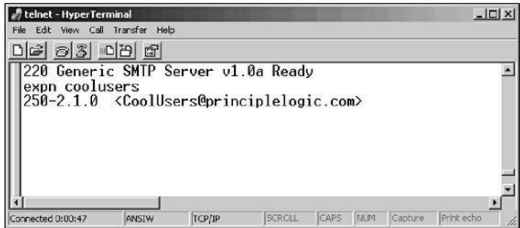
Figure 14.6 : Test d'existence d'une liste de diffusion avec EXPN.
