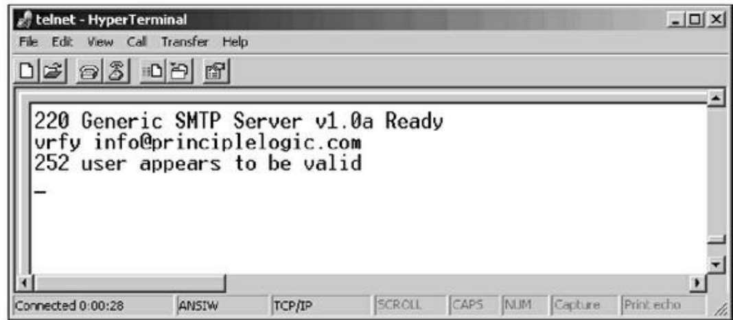
Figure 14.5 : Vérification d'existence d'une adresse de messagerie avec VRFY.
