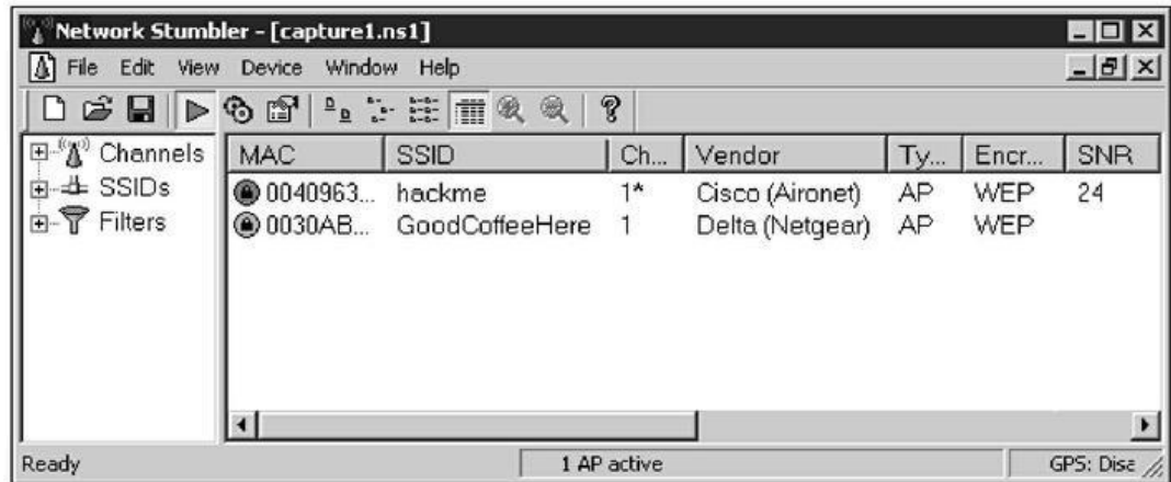
Figure 10.3 : Affichage des détails des points d'arrêt dans NetStumbler.
