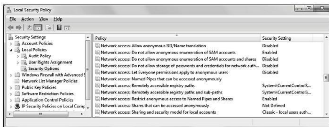
Figure 12.8 : Paramètres de sécurité locale pour interdire les sessions nulles dans Windows 7.
