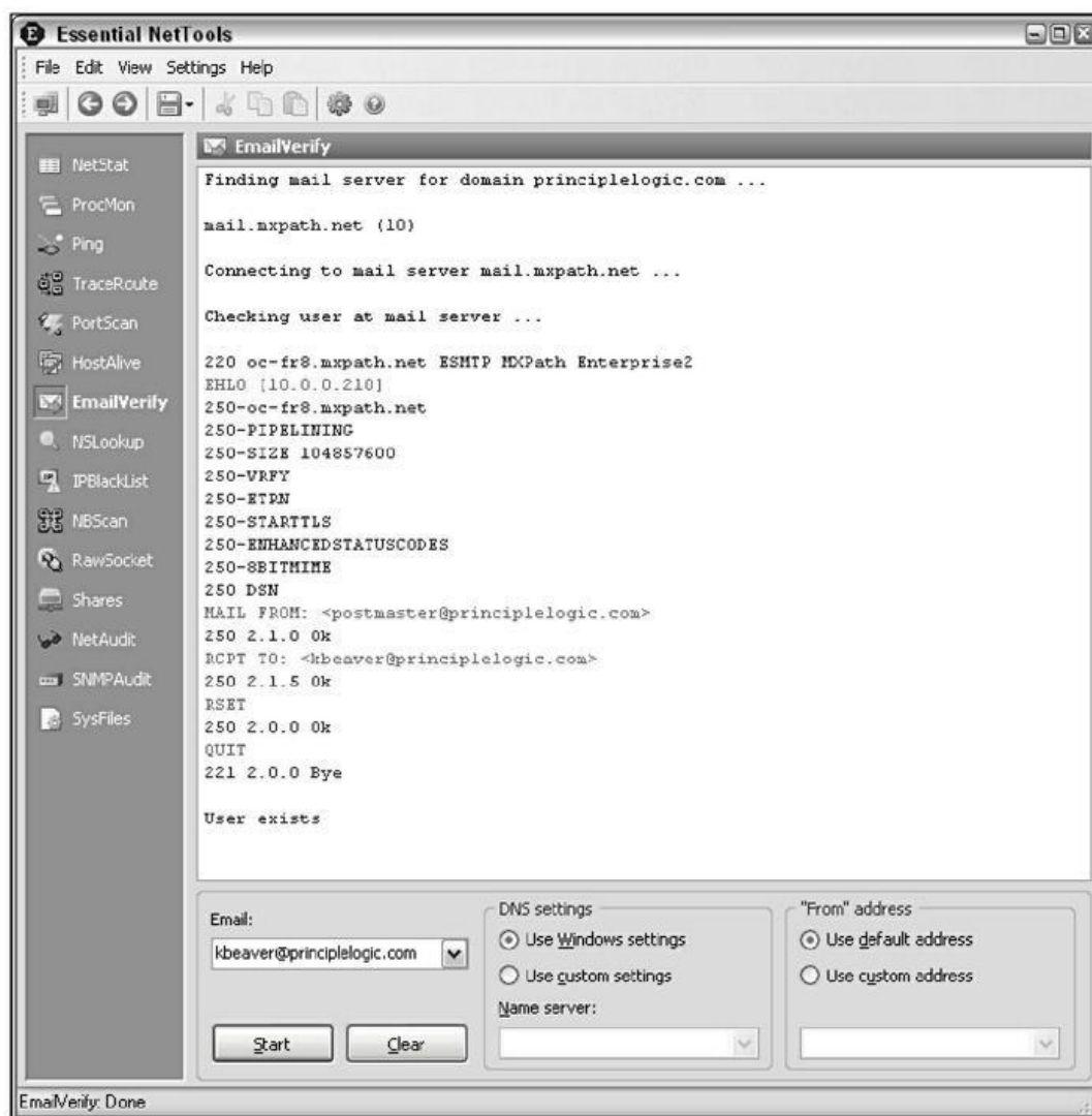
Figure 14.7 : Validation d'une adresse de messagerie avec EmailVerify.
