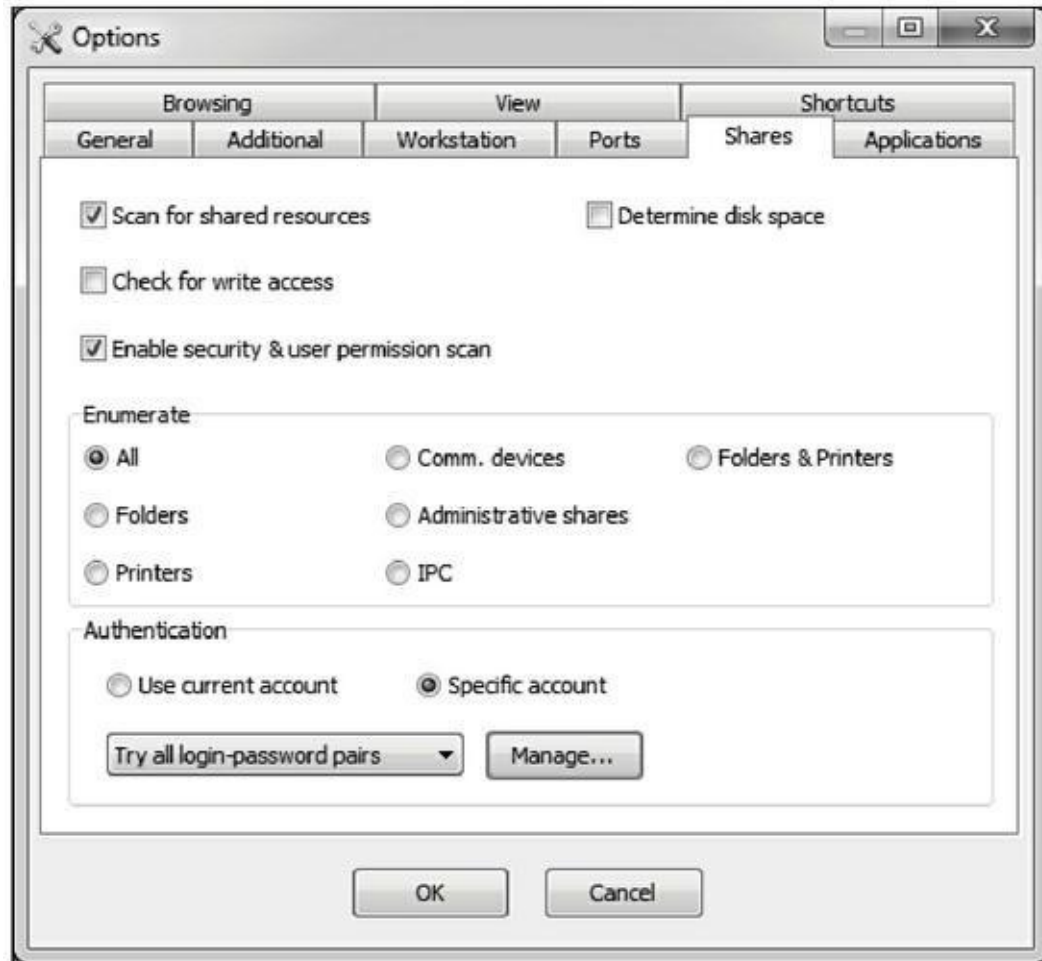
Figure 16.3 : SoftPerfect Network Scanner trouve les partages réseau.
