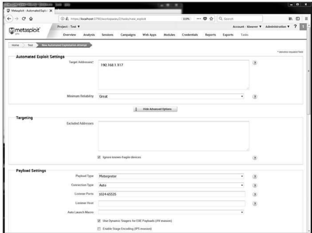
Figure 12.15 : Lancement d'un exploit dans Metasploit Pro à partir de failles découvertes.
