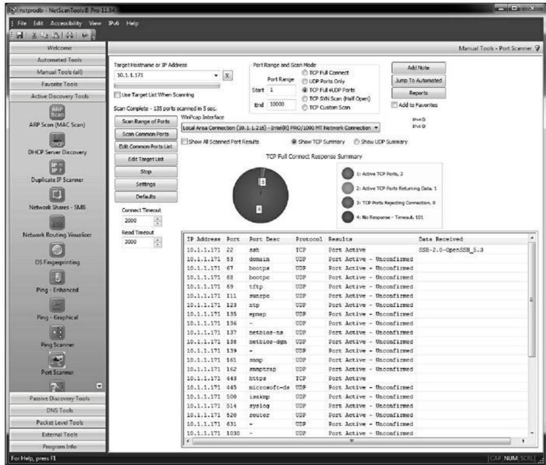
Figure 13.1 : Analyse des ports Linux avec NetScanTools Pro.
