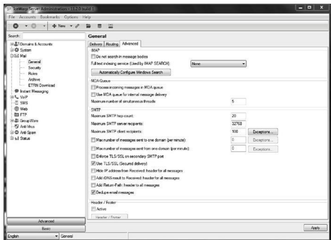
Figure 14.1 : Limitation du nombre de ressources pour les messages entrants.
