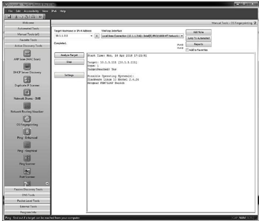
Figure 13.5 : NetScanTools Pro a détecté un Linux Slackware.
