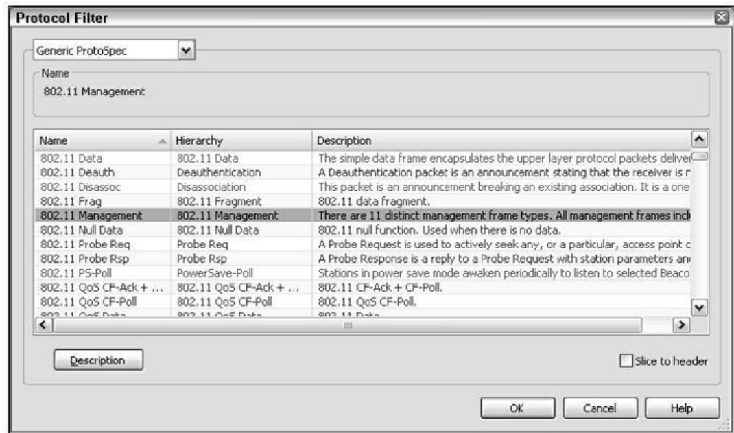
Figure 10.13 : Configuration d'Omnipeek pour détecter les points d'accès qui ne diffusent pas leur SSID.
