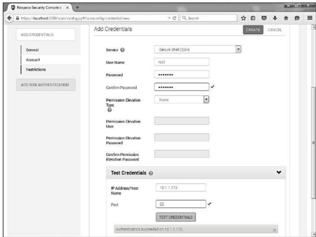
Figure 13.3 : La fonction Test Credentials de Nexpose.
