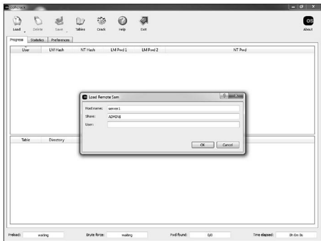
Figure 11.2 : Récupération des valeurs de hachage depuis une base SAM distante avec ophcrack.
