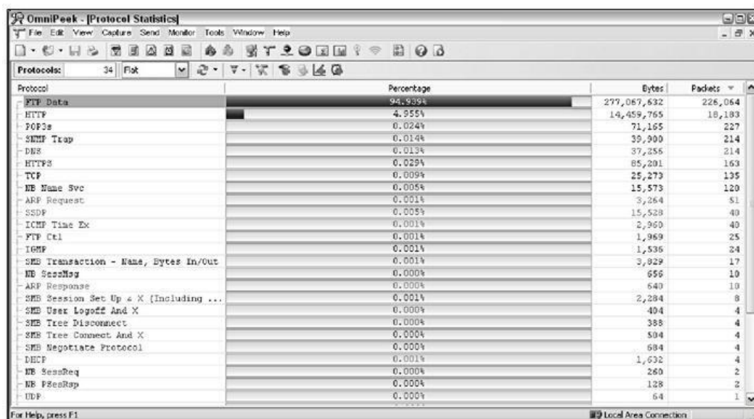
Figure 9.8 : L'outil Omnippeek permet de détecter un serveur FTP illégal.
