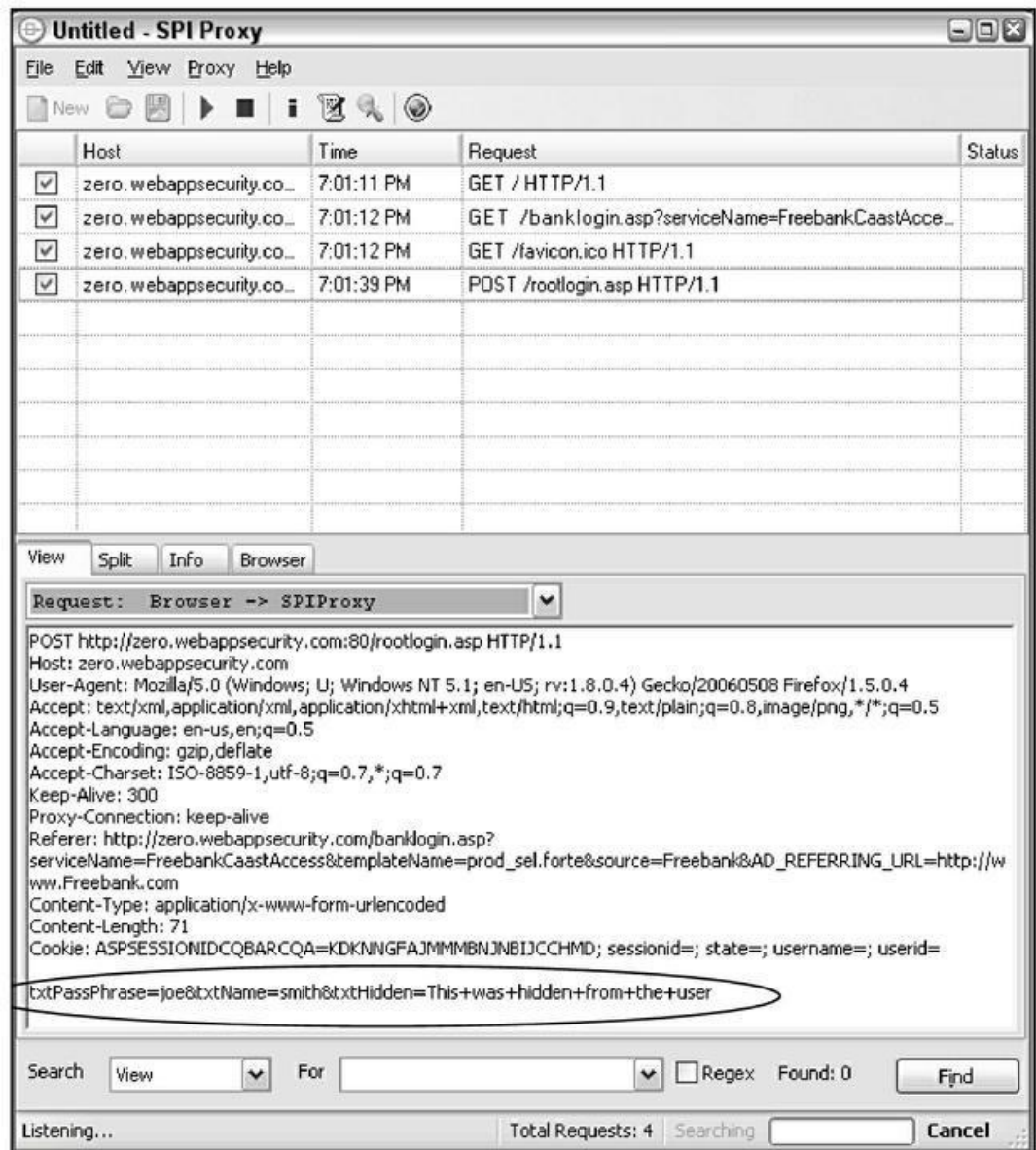
Figure 15.3 : WebInspect trouve et modifie les champs cachés.
