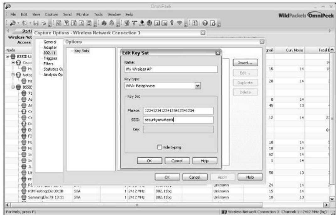
Figure 10.8 : Visualisation du trafic sans fil crypté dans Omnippeek.
