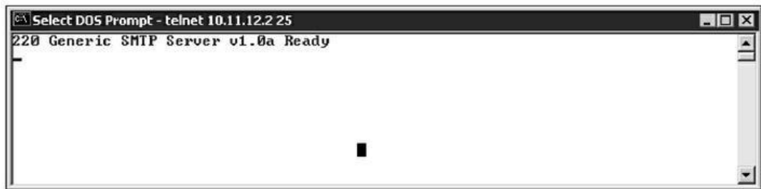
Figure 14.2 : La bannière SMTP montre le numéro de version du serveur.
