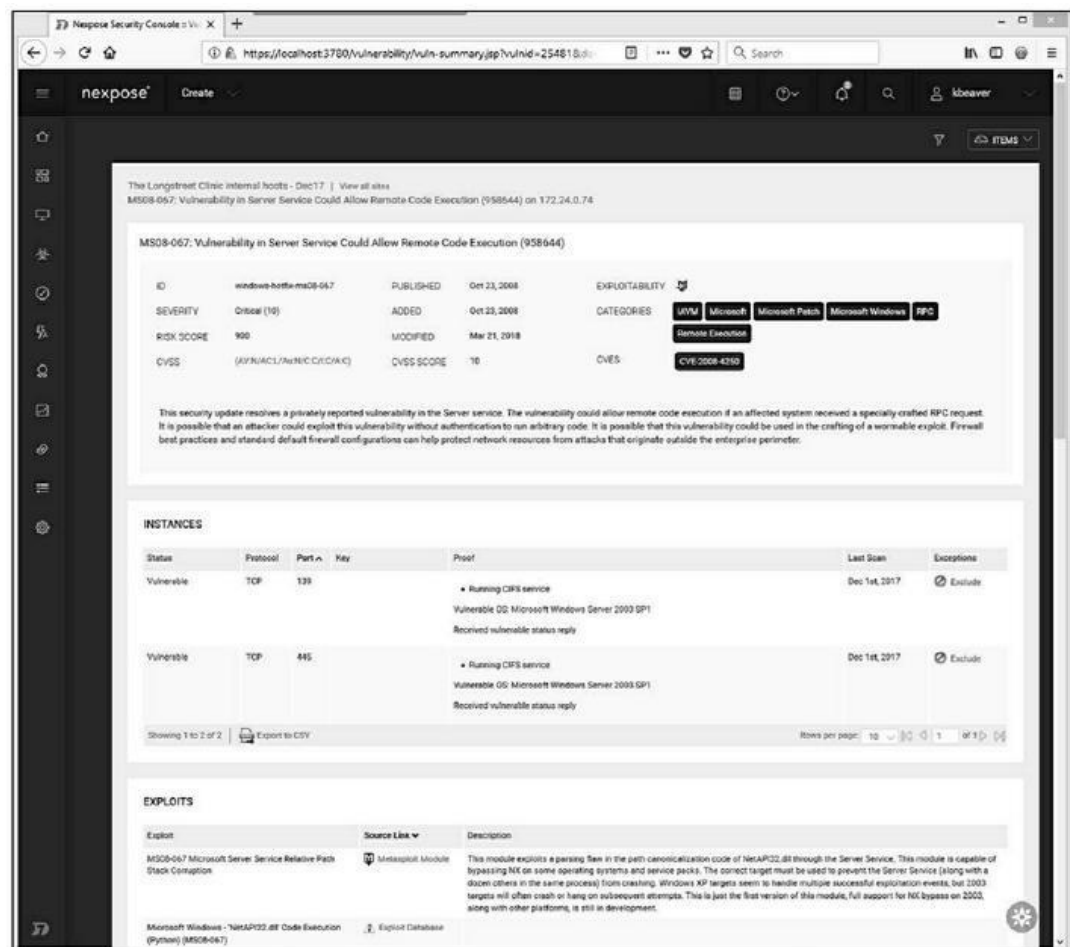
Figure 12.10 : Une faille de correctif trouvée par Nexpose.
