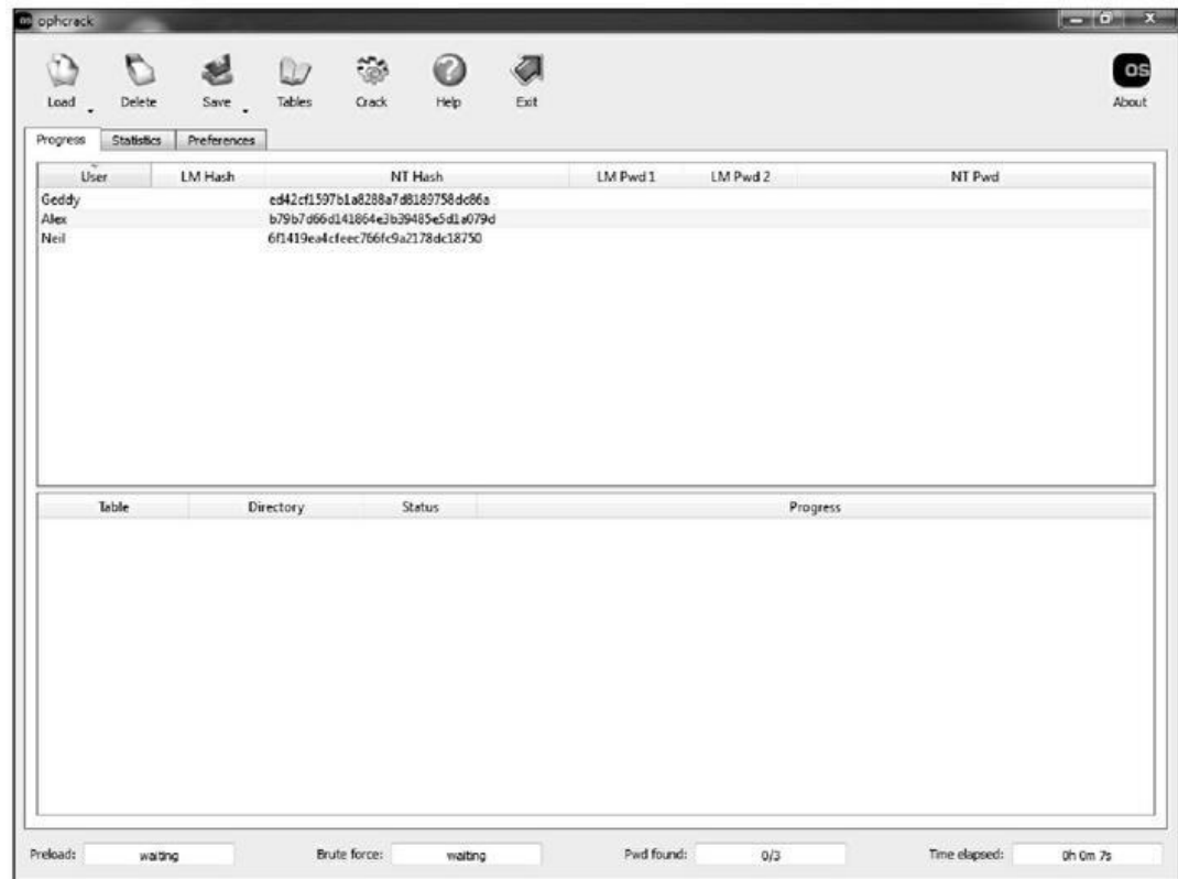
Figure 11.3 : Nom d'utilisateur et valeurs de hachage extraits par ophcrack.
