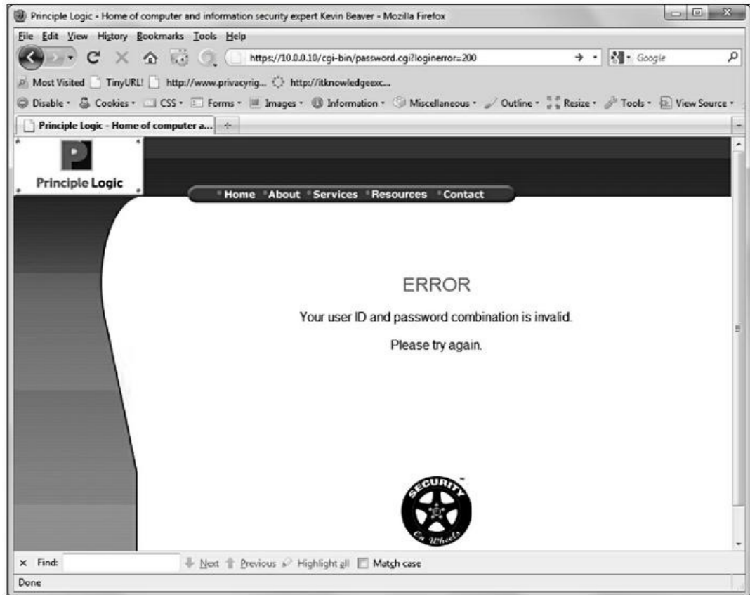
Figure 15. 8 : L'adresse URL montre une autre erreur lorsque c'est le mot de passe qui était invalide.
