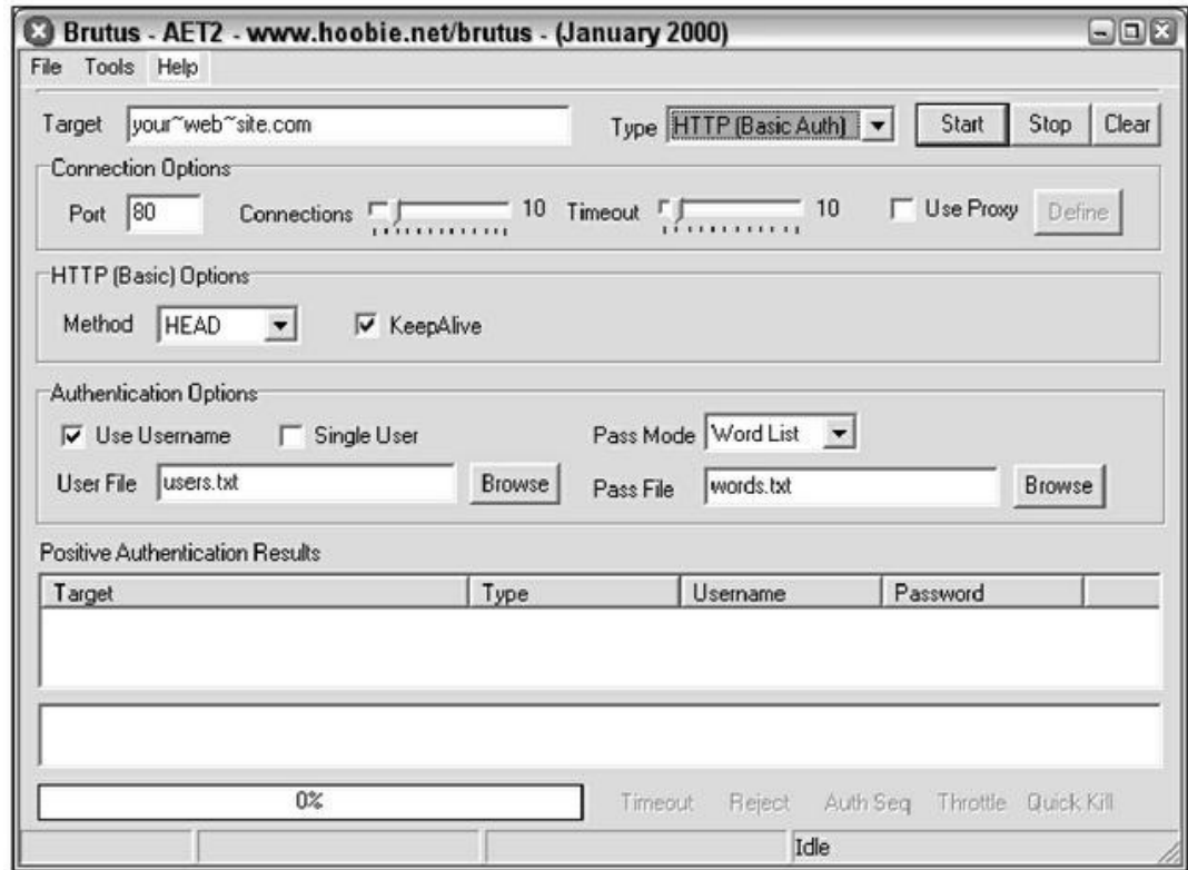
Figure 15.9 : L'outil Brutus teste les mécanismes de login Web fragile.
