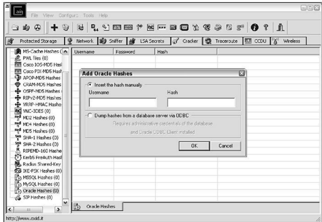
Figure 16.2 : Cain & Abel permet de craquer les mots de passe cryptés d'Oracle.
