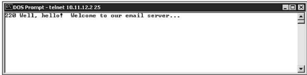
Figure 14.3 : La bannière SMTP n'indique que le numéro de version.
