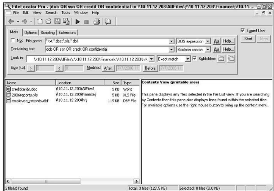
Figure 16.4 : FileLocator Pro permet de trouver du texte sensible dans des partages non protégés.
