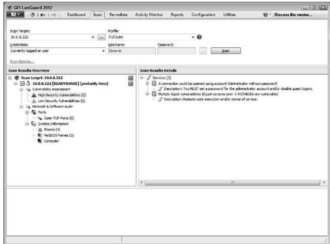
Figure 10.4 : Résultat d'une analyse d'un point d'accès par LanGuard.
