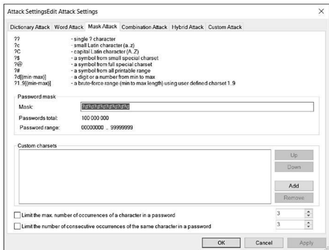
Figure 10.9 : Les options de cassage de mots de passe de l'outil EWSA
