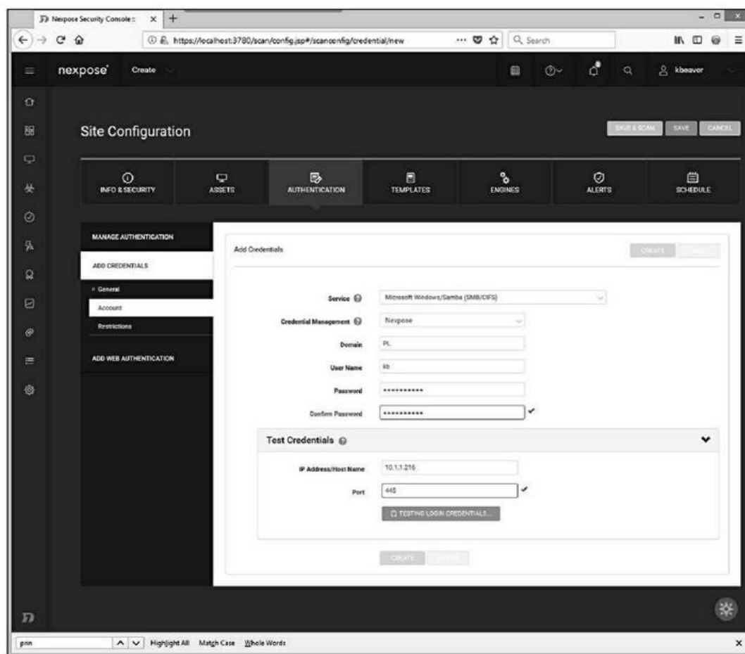
Figure 12.16 : Test des identifiants avant lancement d'une analyse avec Nexpose.
