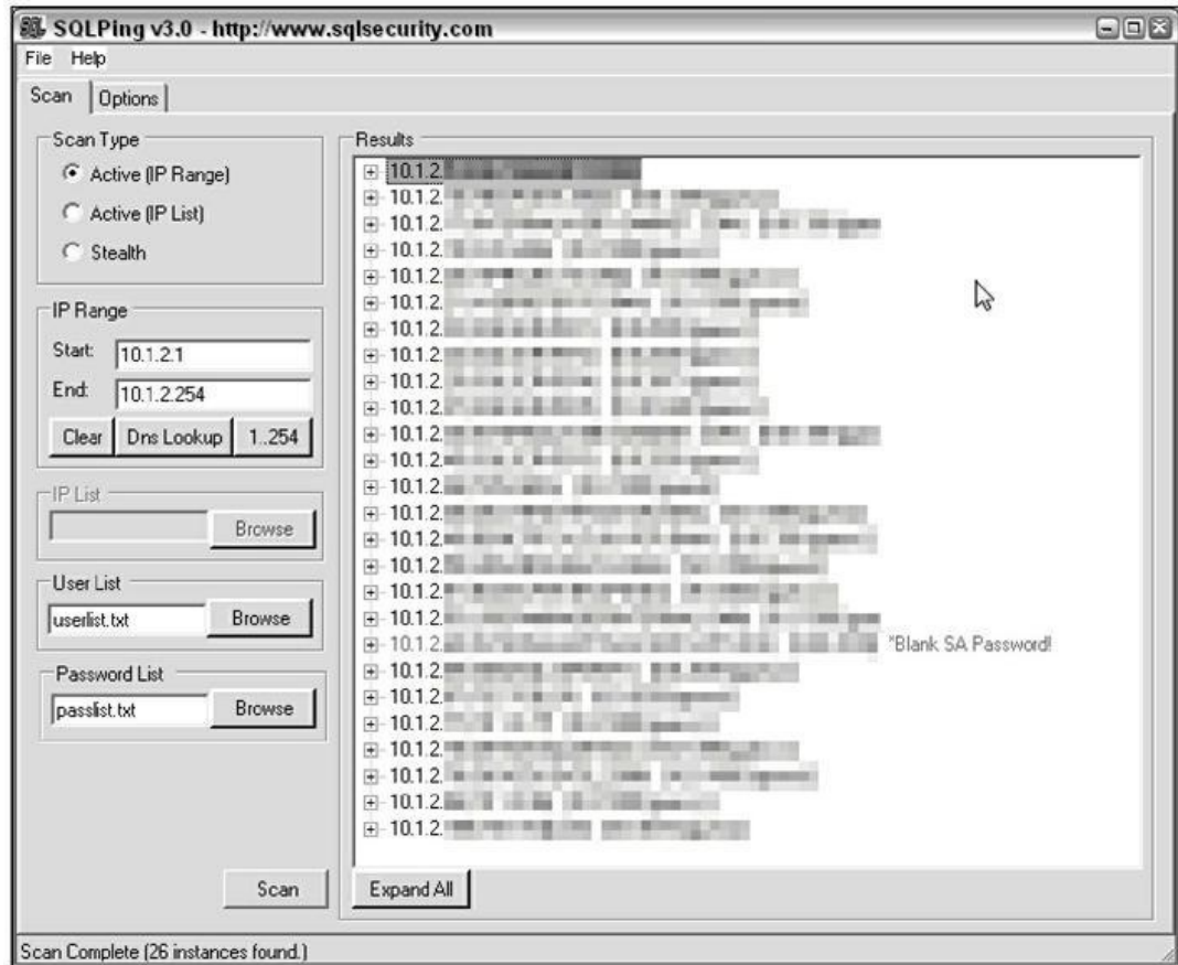
Figure 16.1 : SQLPing3 localise SQL Server et cherche l'absence de mots de passe du compte sa.
