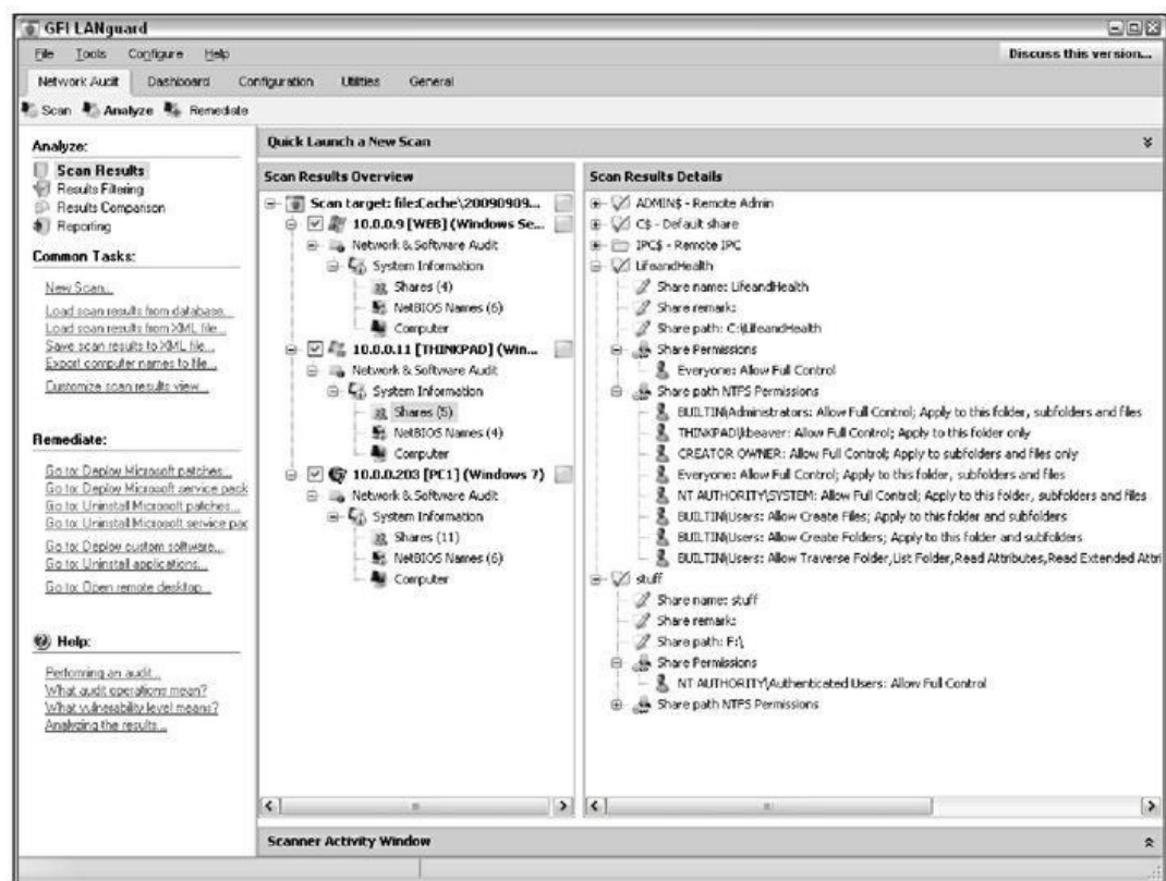
Figure 12.5 : L'outil LanGuard pour analyser les partages Windows.
