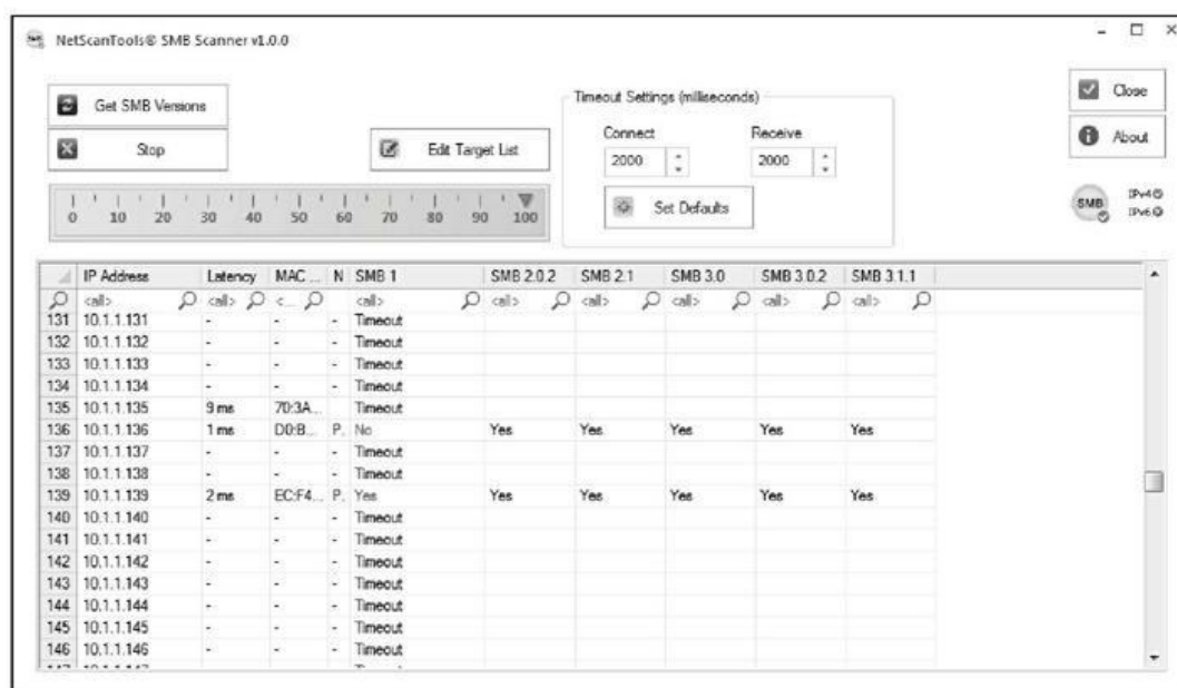
Figure 12.2 : Collecte des versions SMB avec NetScanTools SMB Scanner.
